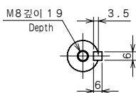
키 부착 Shaft with key
