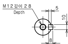
키 부착 Shaft with key
